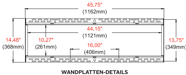
WANDPLATTEN-DETAILS
