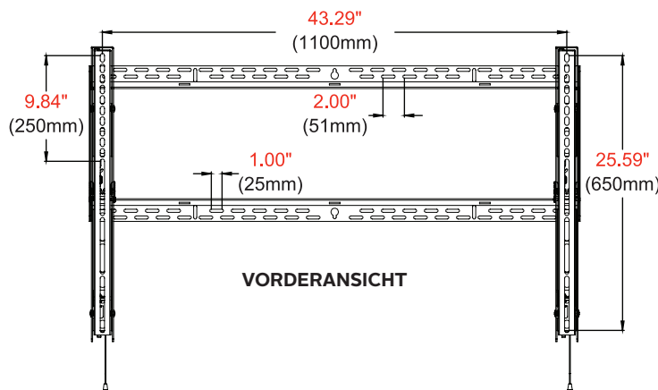
WANDPLATTEN-DETAILS
